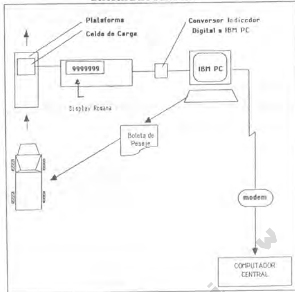
SISTEMA DE PESAJE DE CAMIONES DIAGRAMA GENERAL
